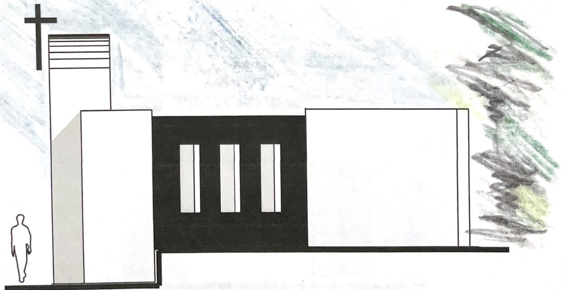
pohled východní 1:100
